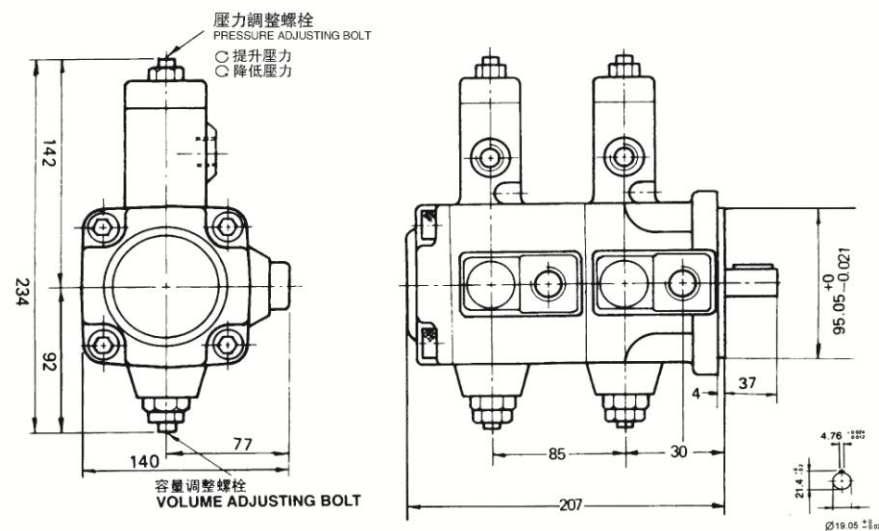
VP-F2323,F2626,F3030,F4040
