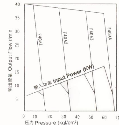
VP-40
