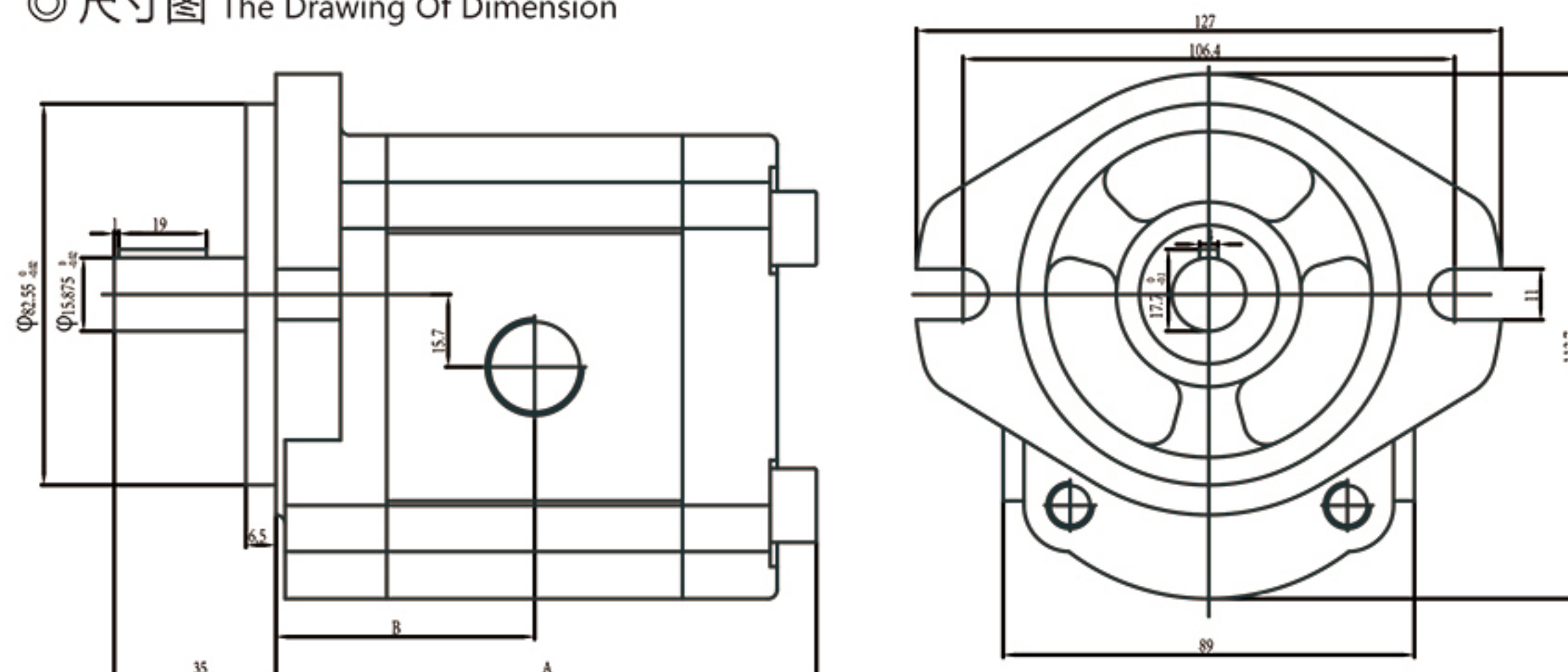
◎ 尺寸 Size
